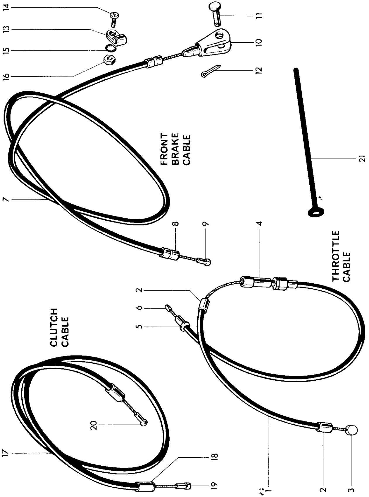
Fig. 25. CONTROL CABLES.
