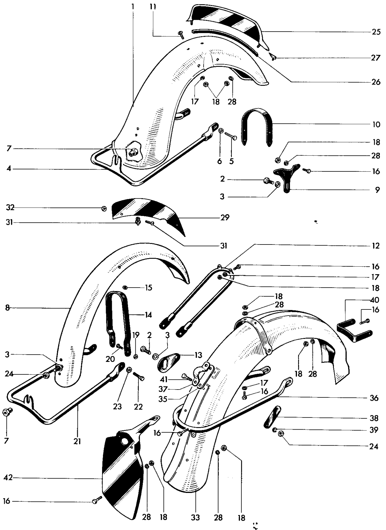
Fig. 20. MUDGUARDS
