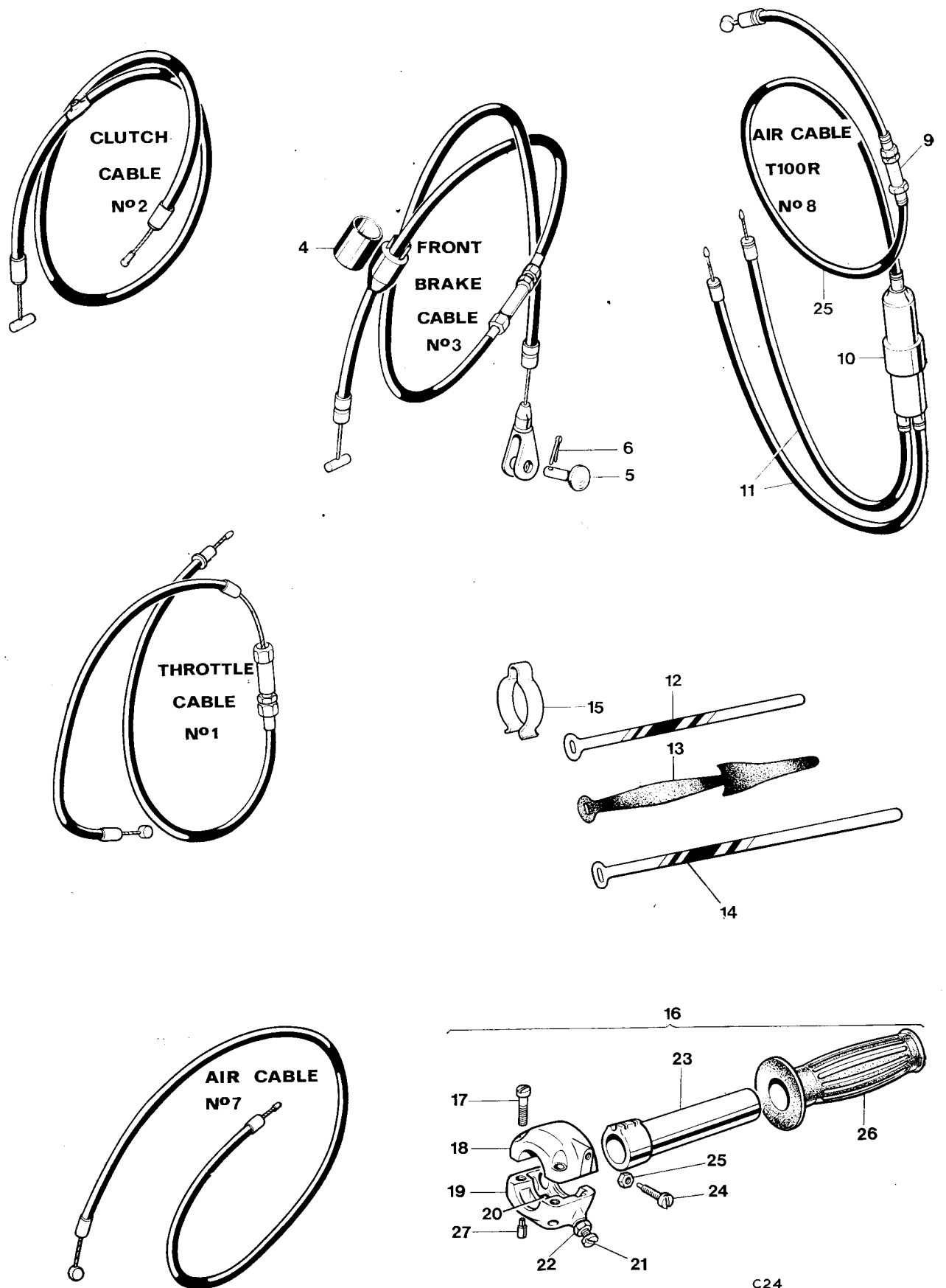
Fig. 31. CONTROL CABLES
