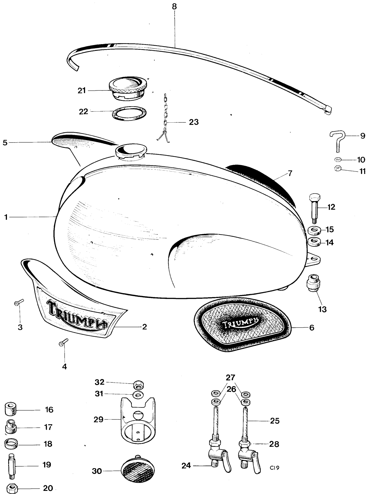
Fig. 27. GAS TANK
