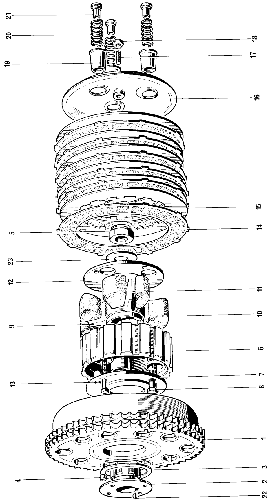
Fig. 13. CLUTCH
