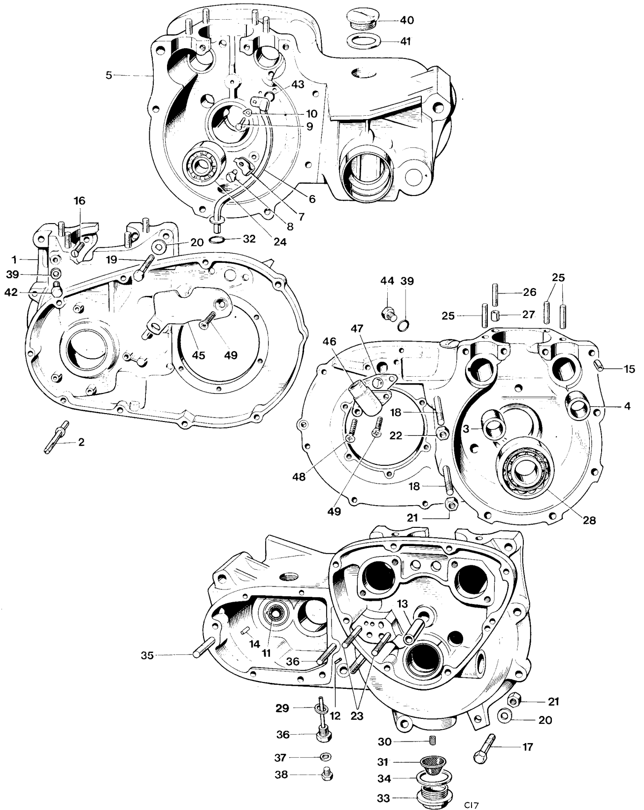
Fig. 2. CRANKCASE
