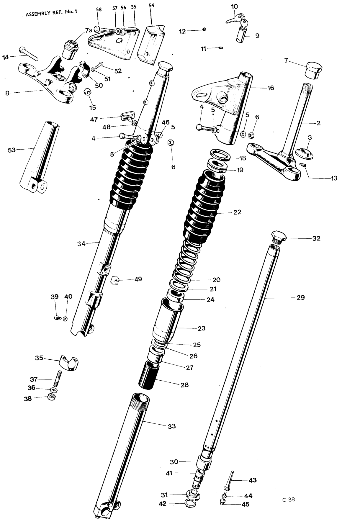
Fig. 20. TELESCOPIC FRONT FORK
