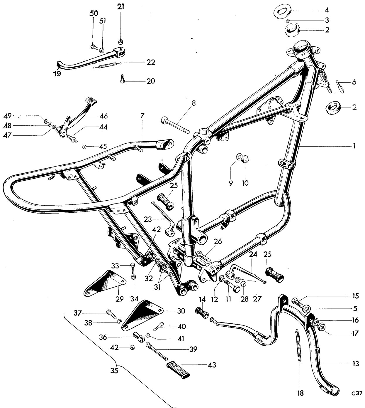
Fig. 18. FRAME
