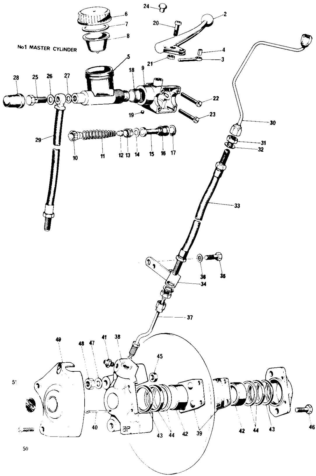
Fig. 23. FRONT BRAKE
