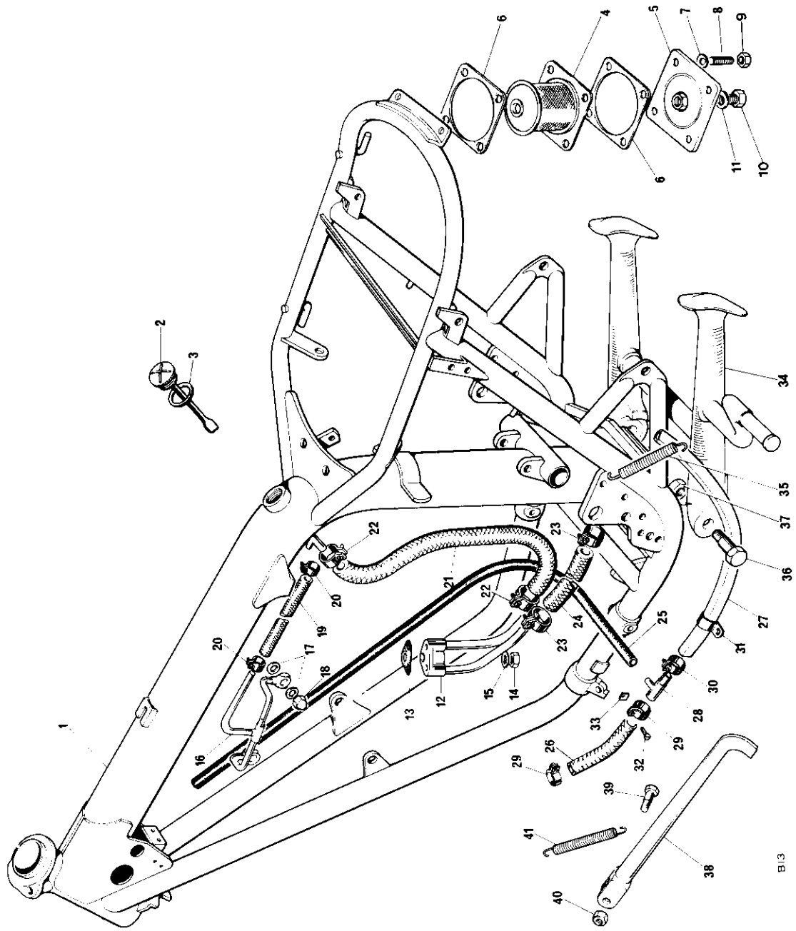
16. FRAME
