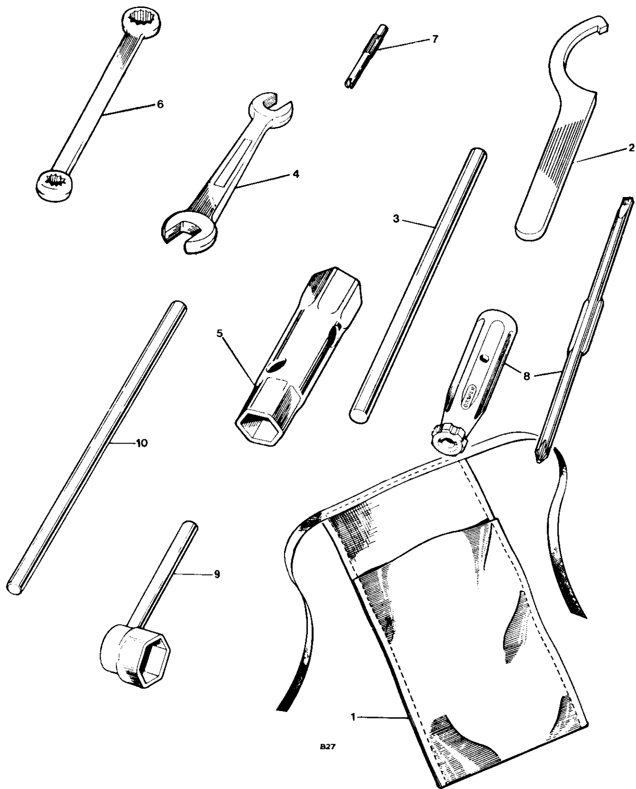
Fig. 31. TOOLKIT
